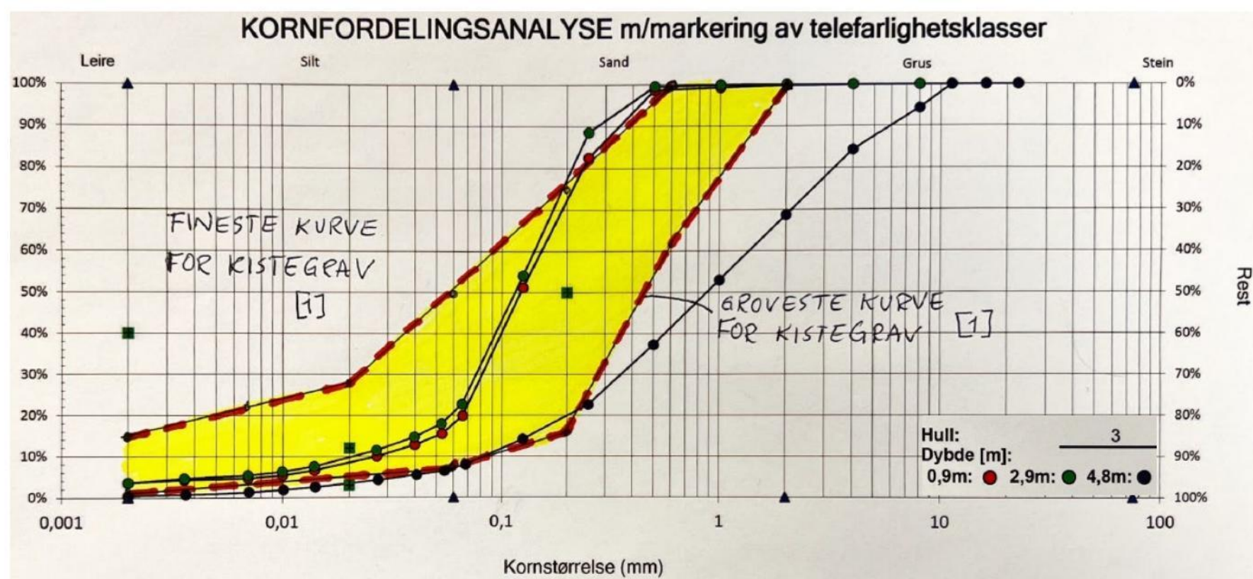
Figur 4. Sammenstilling av utførte korngraderingsanalyser i borepunkt 3
