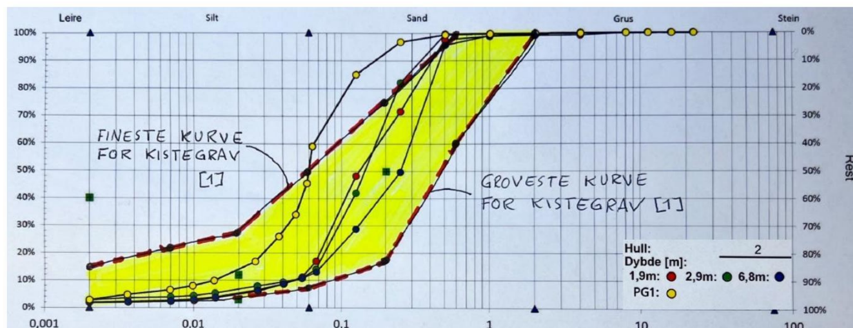
Figur 3. Sammenstilling av utførte korngraderingsanalyser i borepunkt 2
